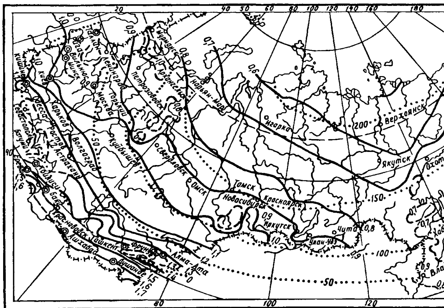
Черт. 3. Климатические коэффициенты для определения величины нагрузки на иловые площадки (сп. линии) и продолжительности периода намораживания на иловых площадках, дни (точечные)
