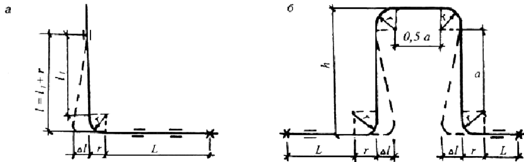
Рисунок 3 - Схемы гнutoго отвода и компенсатора а - отвод; б - компенсатор
