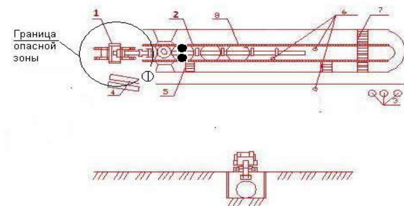
Рис.26. Схема производства работ по укладке стеклопластиковых труб
