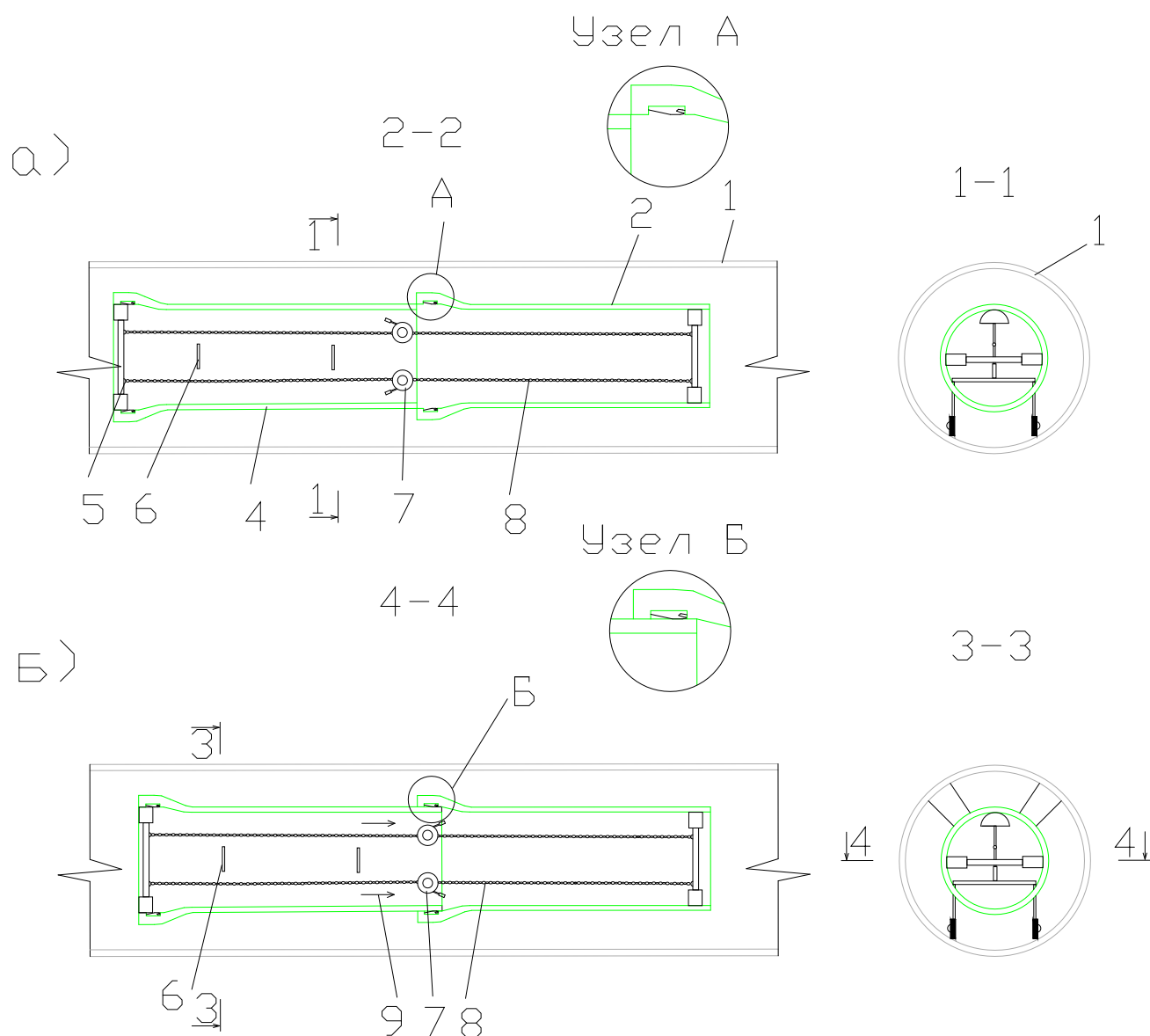
Рис.20 Соединение труб HELYX (соосно)
