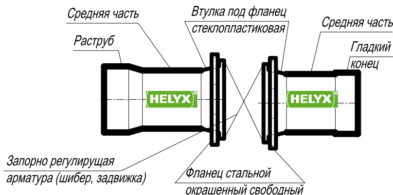
Рис Фланцевое соединение патрубков под фланец с запорно-регулирующей арматурой на стальных свободных фланцах на концах.
