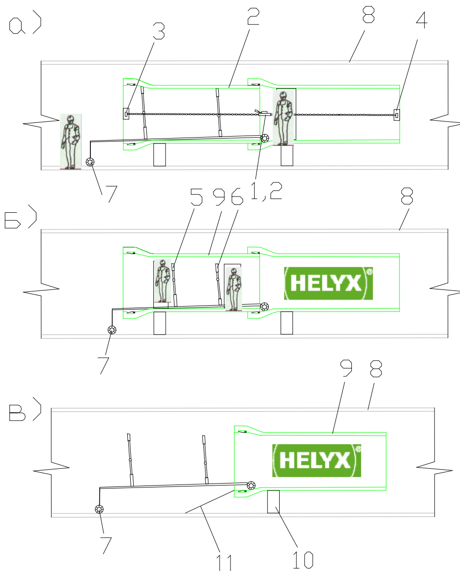
Рис. 22 Снятие монтажной оснастки
