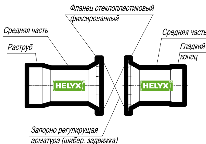
Рис Фланцевое соединение патрубков под фланец с запорно-регулирующей арматурой на стеклопластиковых фиксированных фланцах на концах.
