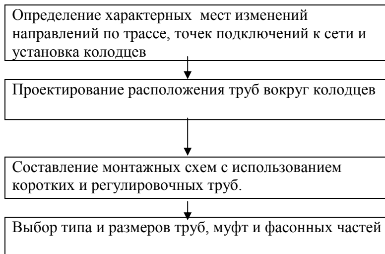
Рис Алгоритм проектирования с применением стеклопластиковых труб.
