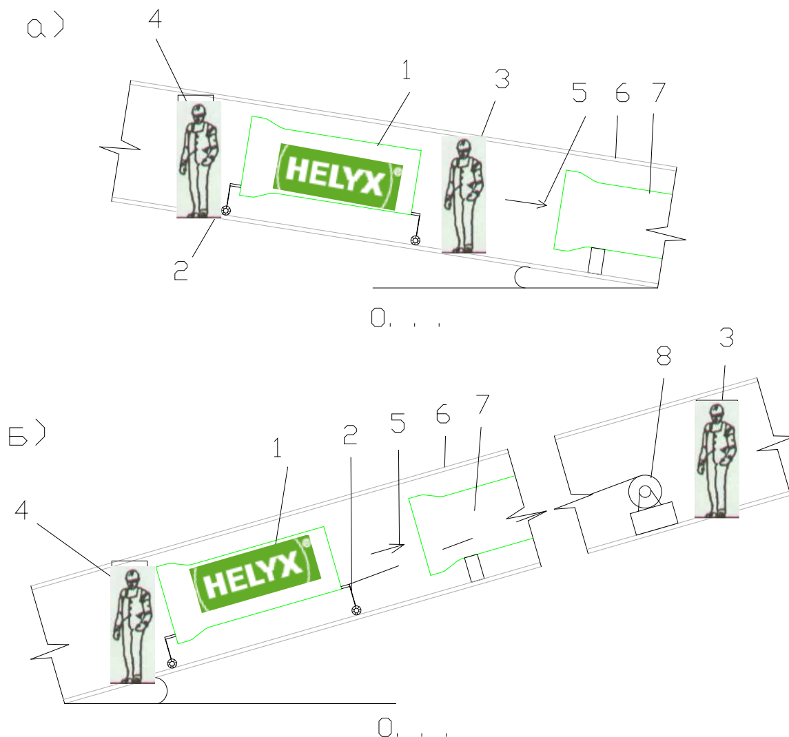
Рис. 17 Транспортировка трубы HELYX к месту установки
