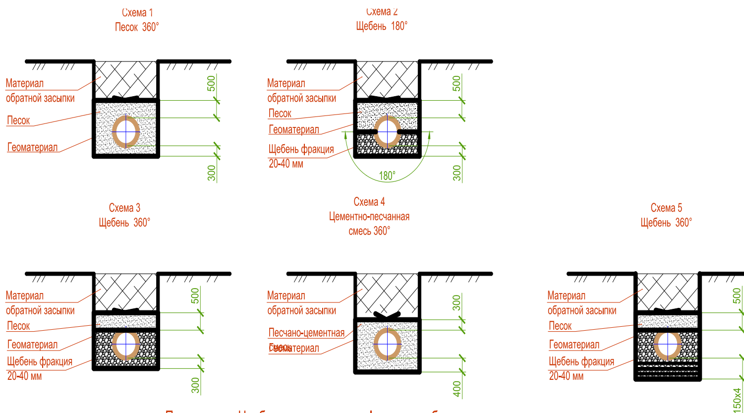
Рис.6. Схемы типов оснований из разных материалов
