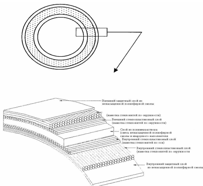
Рис.1 Разрез стеклопластиковой трубы Helyx.
