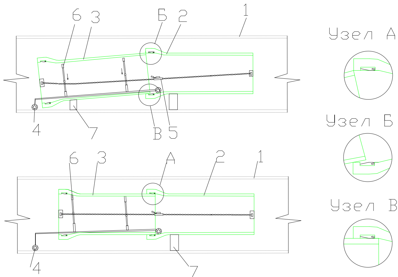
Рис.21 Установка труб HELYX с изменением уклона
