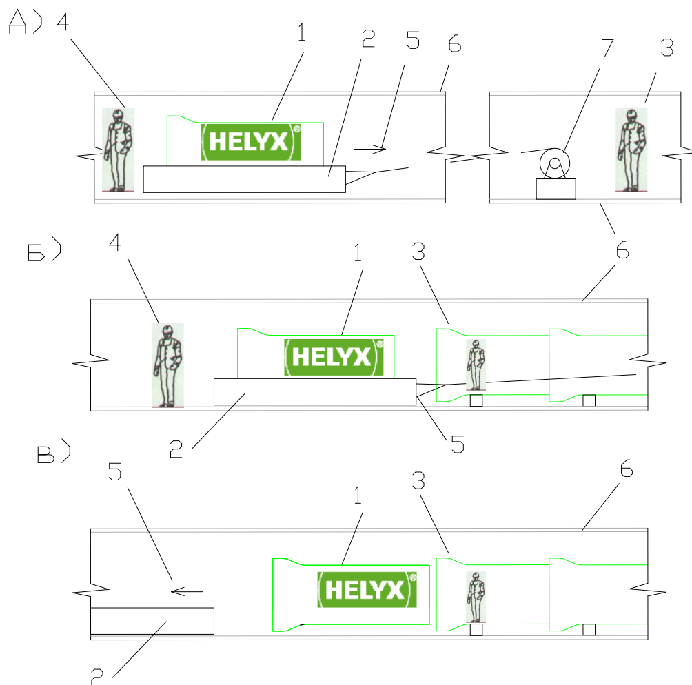
Рис. 17 Транспортировка трубы HELYX к месту установки с использованием лебедки
