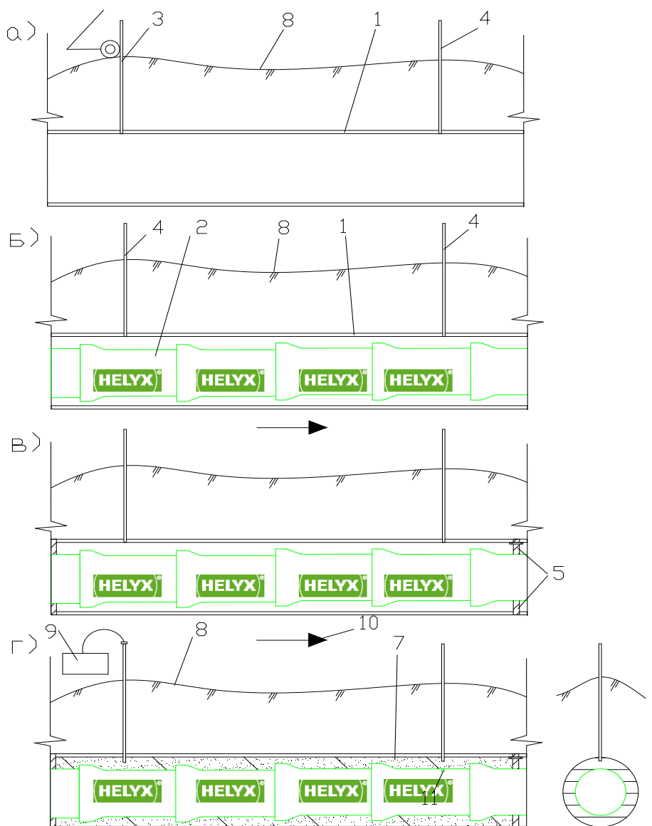
Рис. 23 Заполнение межтрубного пространства цементно-песчаным раствором (1 способ)
