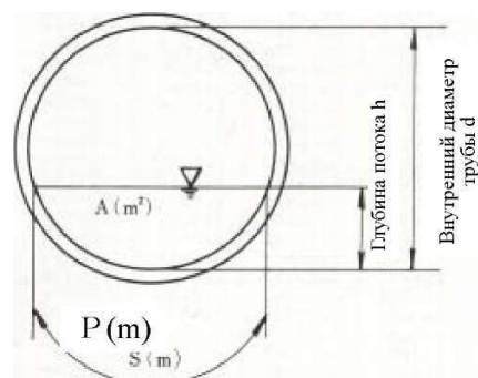
Рис 2. Сечение трубопровода
