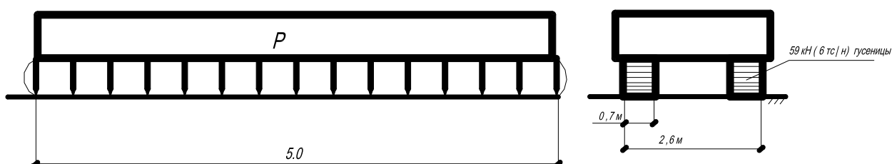
Рис Гусеничная нагрузка от (одной машины) НГ-60 общим весом 588 кН (60 тс.)
