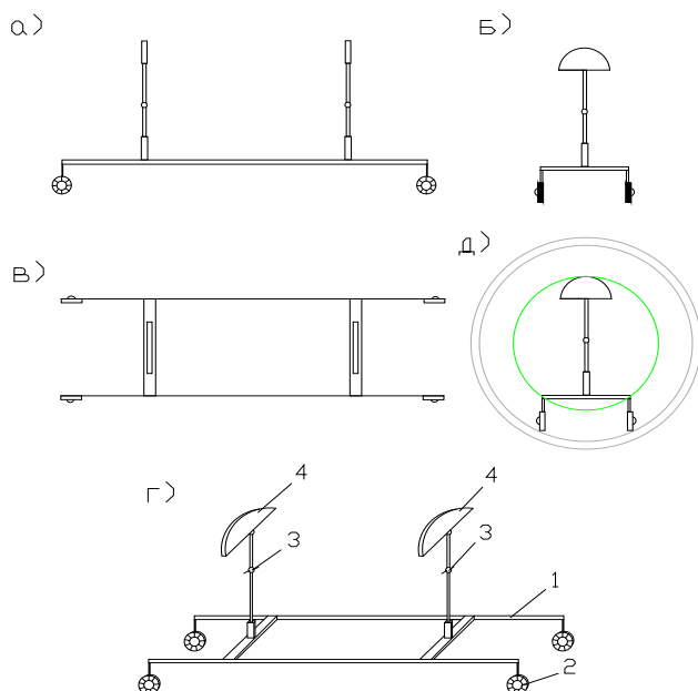
Рис. 15 Тележка для транспортировки и установки труб а) вид спереди б) вид сбоку, в) вид сверху г) пространственная модель д) вид тележки в трубе 1 – металлическая труба 2 – колеса на пневмоходу 3 – реечный домкрат усилием 2т 4 – упоры
