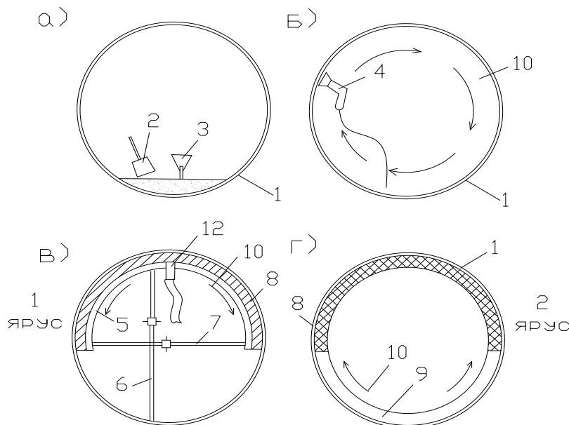
Рис. 14 Подготовка существующей ж/б трубы к санации
