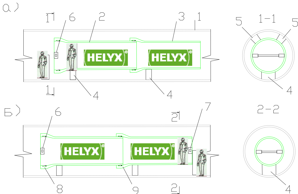
Рис.19 Установка монтажных распорок
