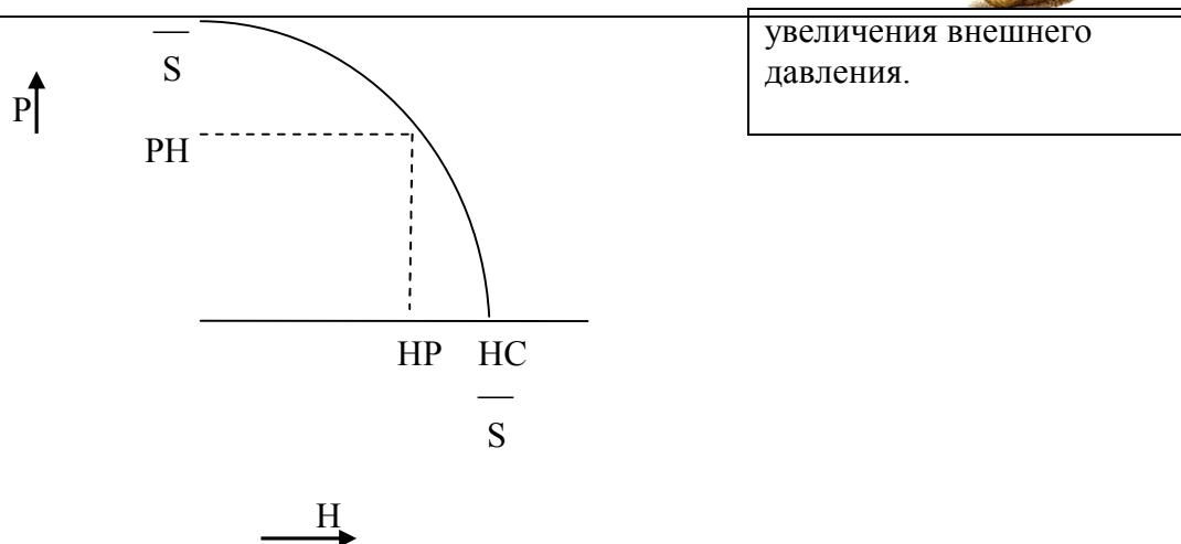
Рис. 5. Зависимость допустимого гидравлического давления от линейной нагрузки
