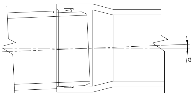
Рис 12. Угол изгиба (угловое смещение) в соединении
