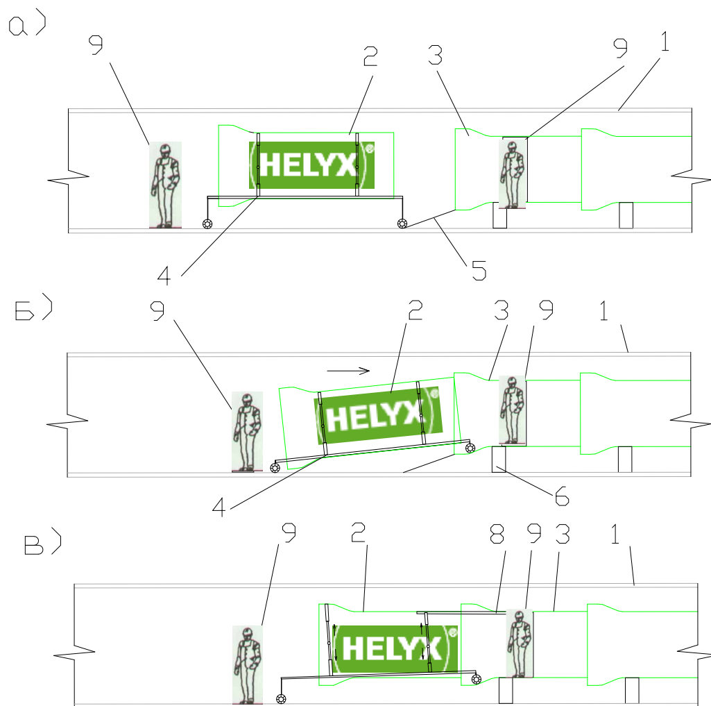
Рис. 18 Установка трубы на месте монтажа с использованием тележки
