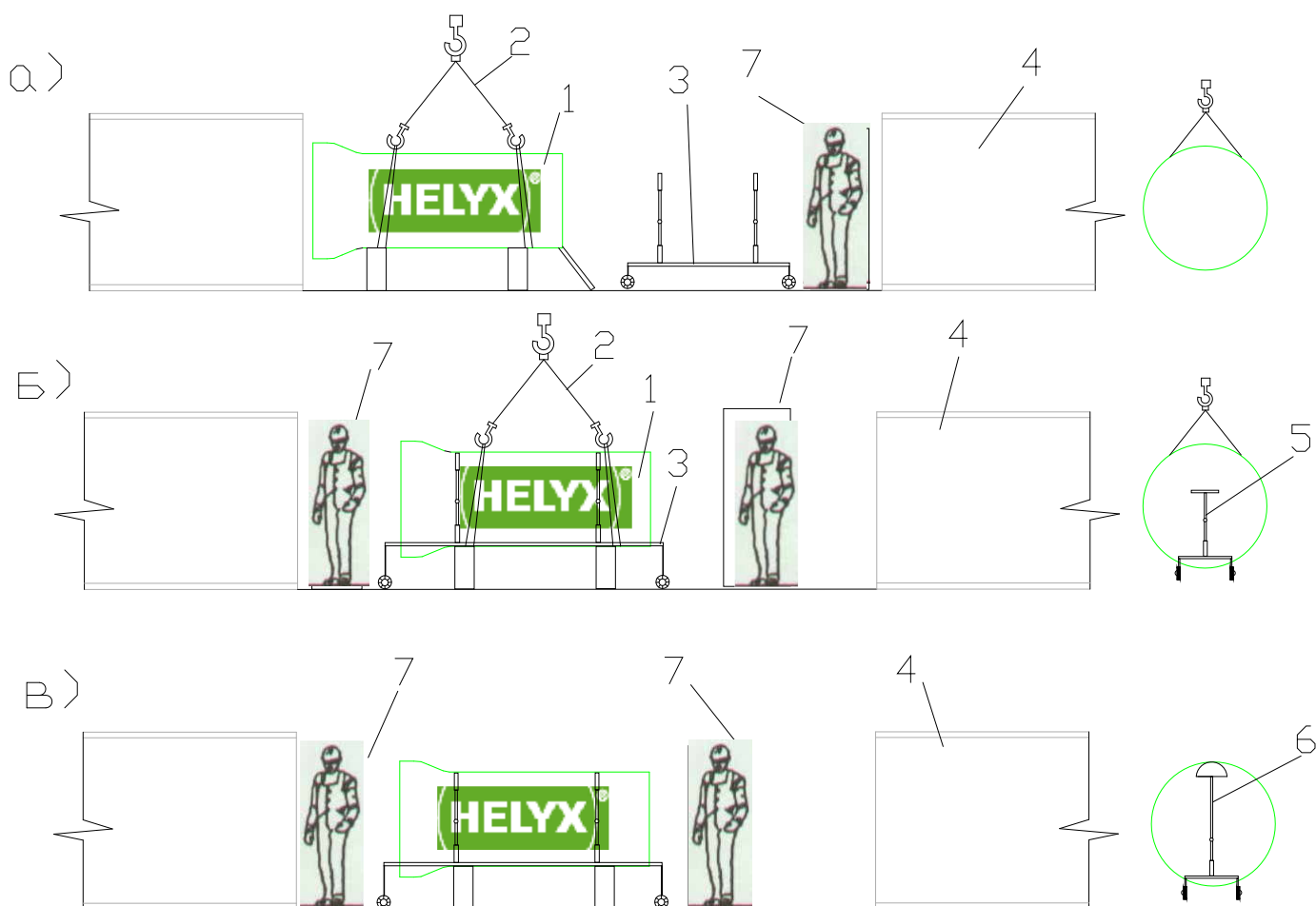
Рис.16 Установка трубы HELYX на тележку
