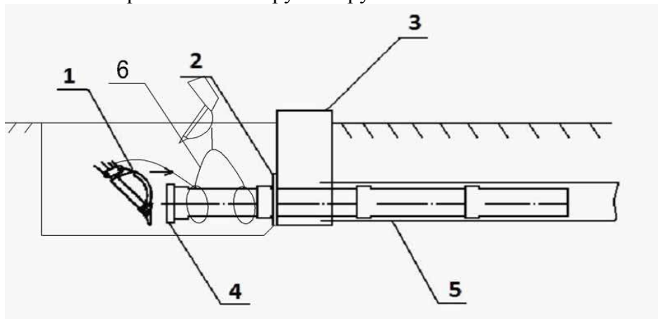
Способ протаскивания труба в трубе
