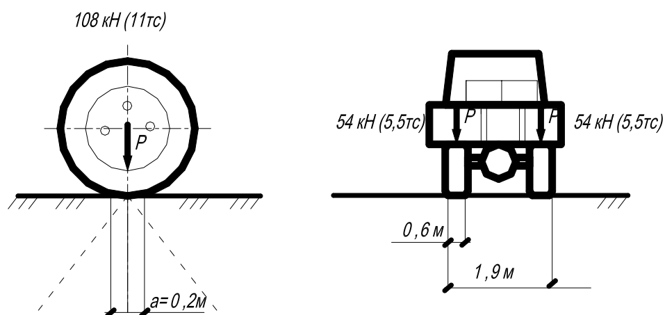
Рис Колесная нагрузка от одноосной тележки с давлением 108 кН (11тс).
