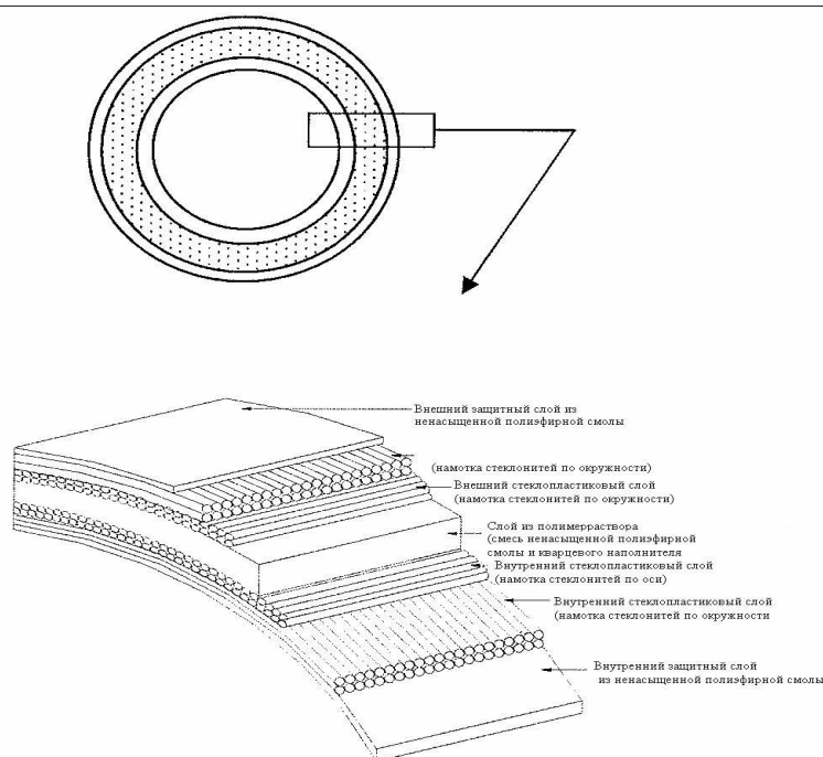
Рис.1 Разрез стеклопластиковой трубы Helyx.
