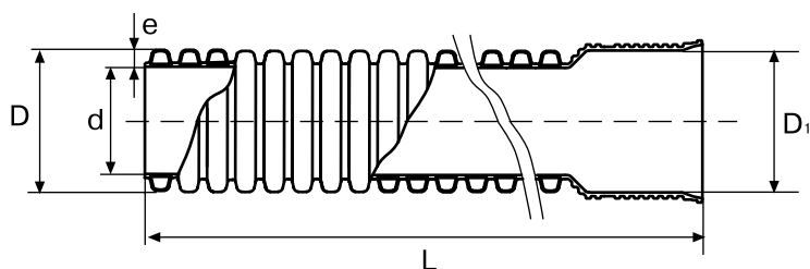
Труба ИКАПЛАСТ исп. 2 (с уменьшенной высотой гофра в месте соединения с раструбом)
