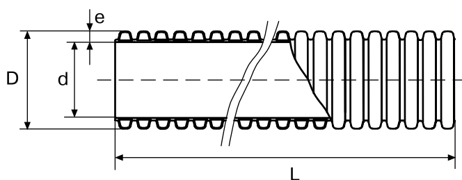
ПП гофрированная труба без раструба
