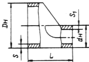
Эксцентрический переход
