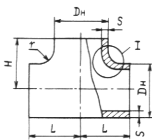
Равнопроходной тройник
