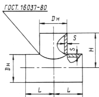
Равнопроходной тройник
