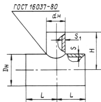
Переходной тройник
