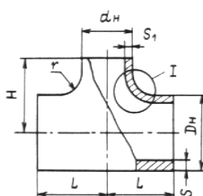
Переходной тройник
