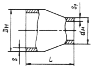
Концентрический переход
