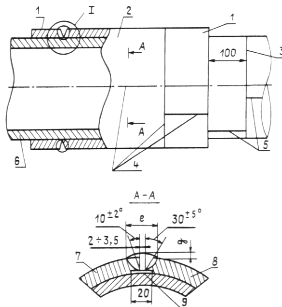
Рис. 7.2. Схема монтажа и сборки муфты с технологическими кольцами:
