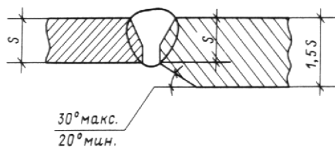
Рис. 11. 1. Конструктивные размеры разделки кромок и сварных швов разнотолщинных труб (до 1,5 толщины стенки)
