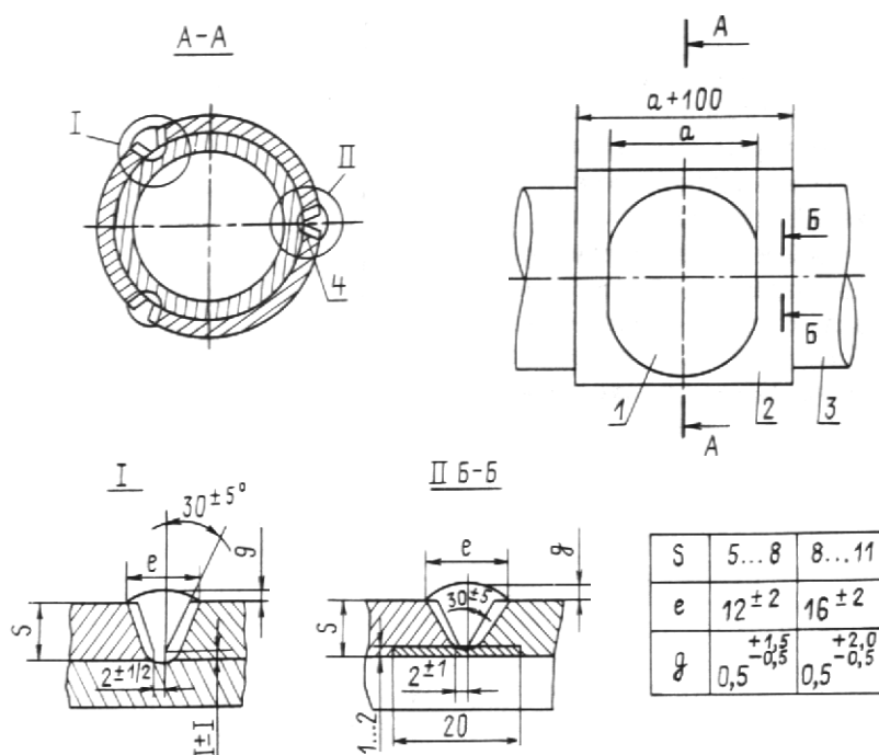
Рис. 7.1. Схема монтажа заплаты с технологическими сегментами: 1 — заплата; 2 — технологические элементы; 3 — труба; 4 — прокладка
