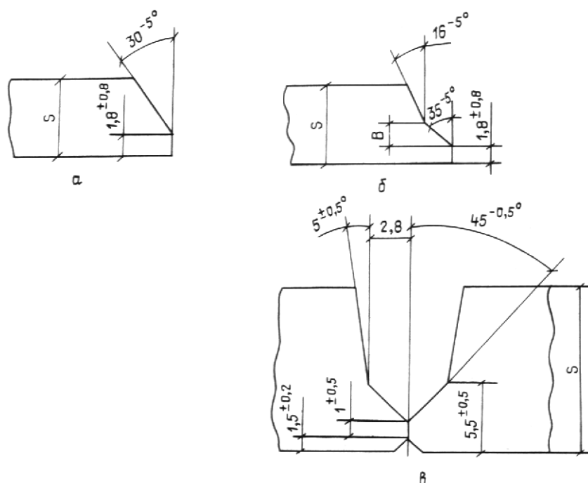
Рис. 8.1. Типы разделки кромок труб для ручной дуговой сварки, односторонней автоматической сварки под флюсом, автоматической дуговой сварки порошковой проволокой с принудительным формированием, полуавтоматической сварки в защитных газах: а — для труб D 57-1420 мм с толщиной стенки до 16 мм; б — для труб D 273-1420 мм с толщиной стенки более 15 мм; в — для автоматической сварки труб в защитных газах
