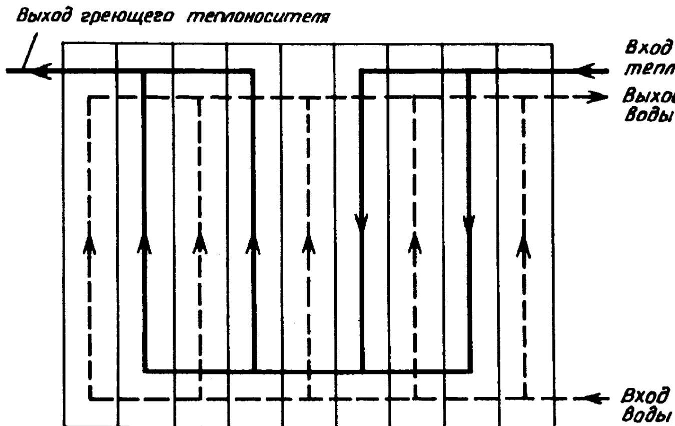
Рис. 2. Несимметричная компоновка пластинчатого водоподогревателя, обозначение Сх (2 + 2)/5"
