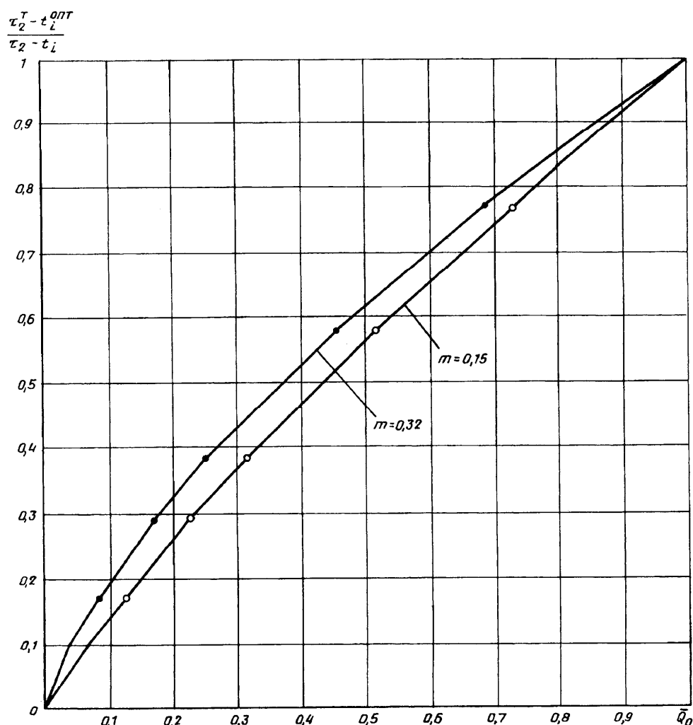
Рис. 3. Графики изменения температурного критерия системы отопления по температуре воды в обратном трубопроводе \frac{\tau_2^T - t_i^{опт}}{\tau_2 - t_i} при постоянной циркуляции воды в системе
