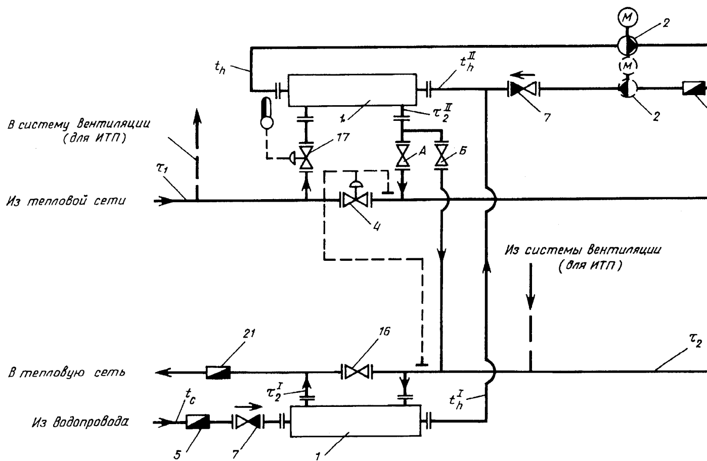
Рис. 8. Двухступенчатая схема присоединения водоподогревателей горячего водоснабжения с зависимым присоединением систем отопления при отсутствии регуляторов расхода теплоты на отопление в ЦТП и ИТП 1 — 21 — см. рис. 1—4
