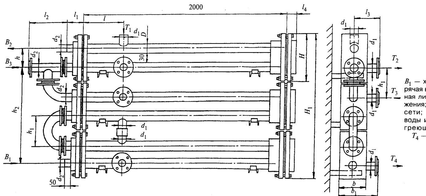
Основные технические характеристики водоподогревателей блочного типа для ИТП (установка из 3 бл.
