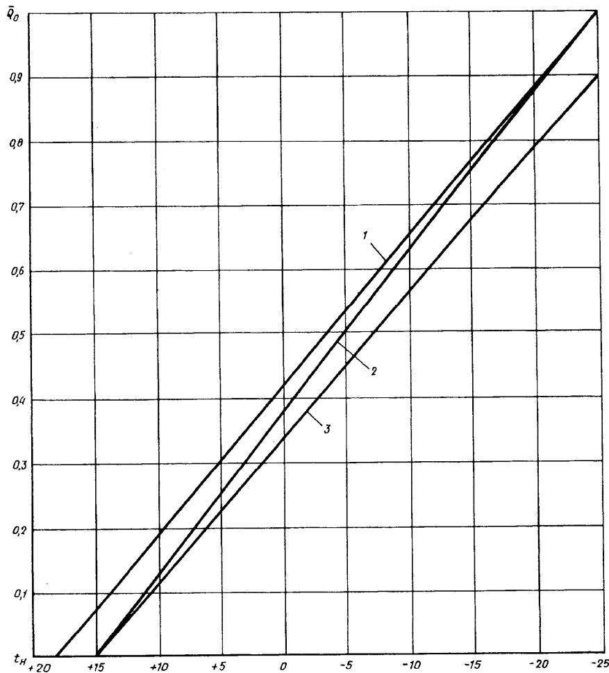
Рис. 1. Графики относительного изменения теплового потока на отопление \bar{Q}_o в зависимости от наружной температуры t_o для разного типа потребителей и способов авторегулирования
